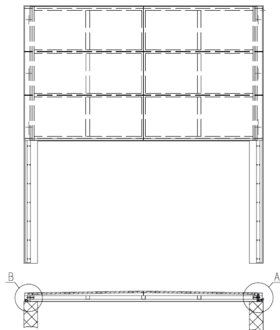
Couvercle de regard ROMAG du type S13
