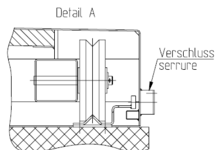
Couvercle de regard ROMAG du type S13 ; détail A
