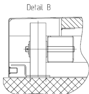
Couvercle de regard ROMAG du type S13 ; détail B
