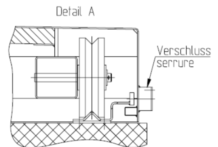
Schachtabdeckung S13; Detail A
