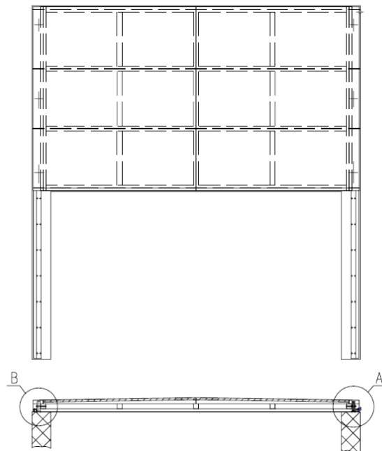
Schachtabdeckung ROMAG Typ S13
