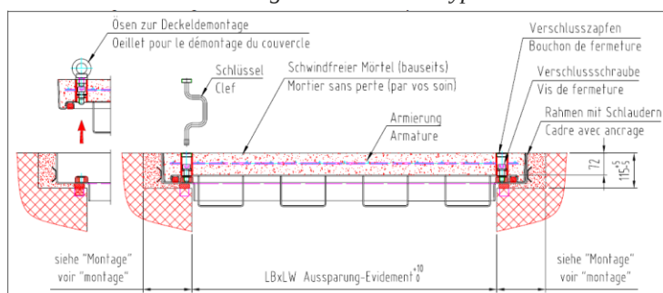
Couvercle de regard ROMAG du type S16
