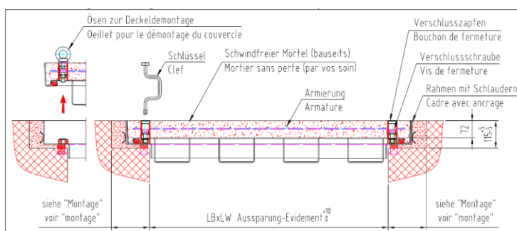
Schachtabdeckung ROMAG Typ S16
