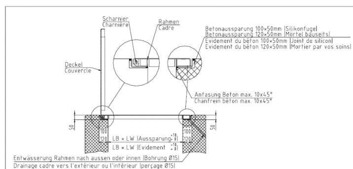
Couvercle de regard ROMAG du type S1b
