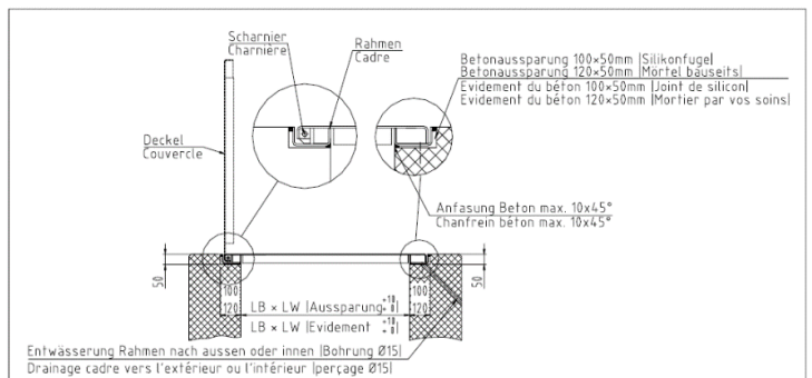
Schachtabdeckung ROMAG Typ S1b
