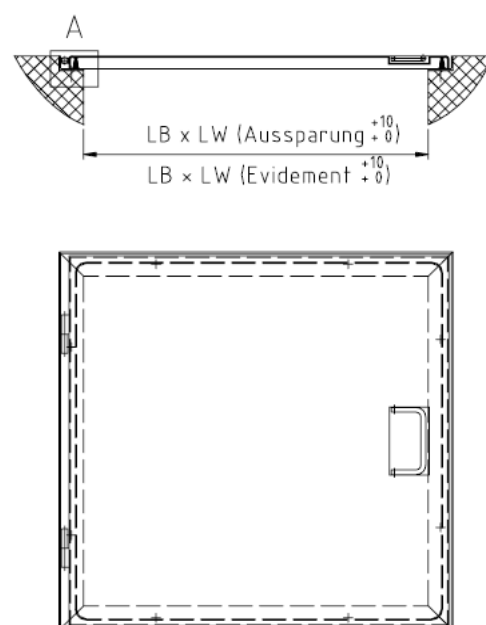
Couvercle de regard étanche aux odeurs ROMAG du type S24b
